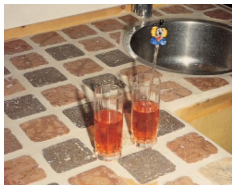
Exemple de collage et de jointoiement d'un plan de travail de cuisine
